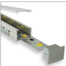
Aufbauprofile
